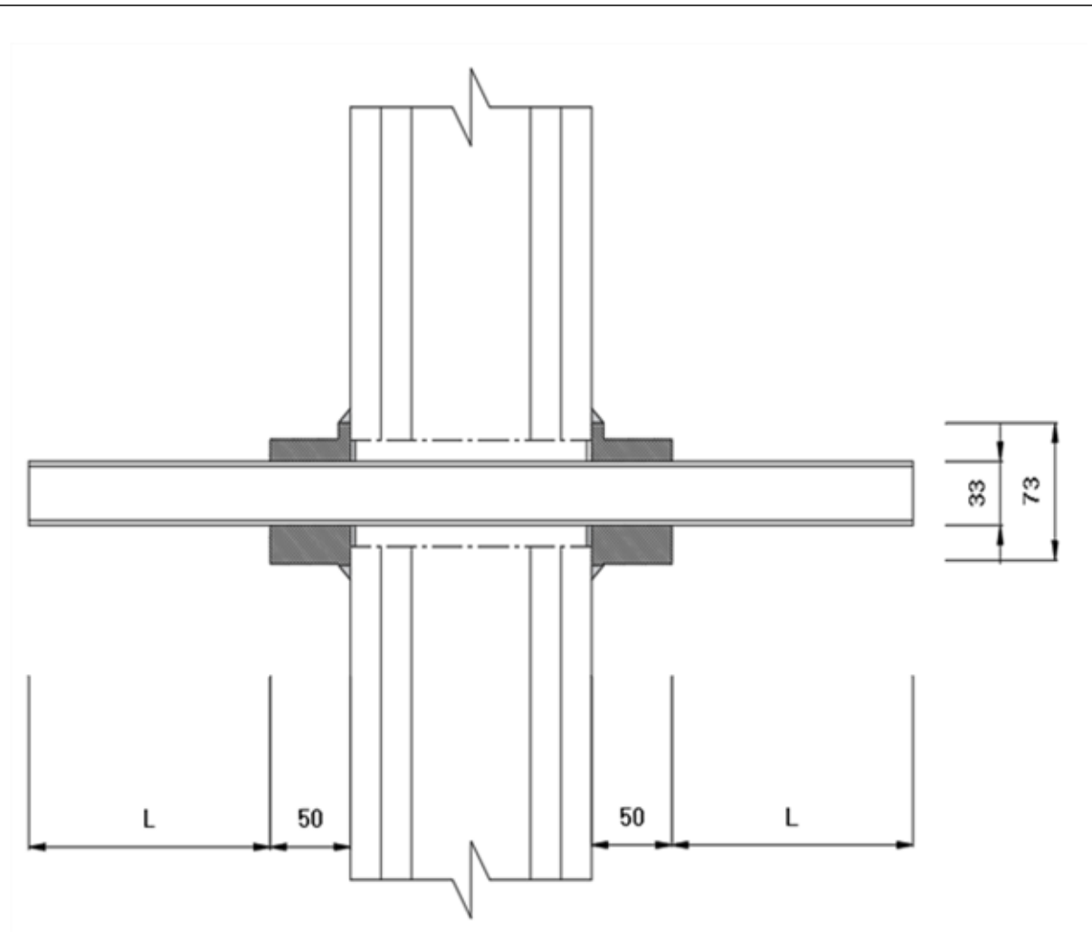
(수직 단면도 (A-A))
