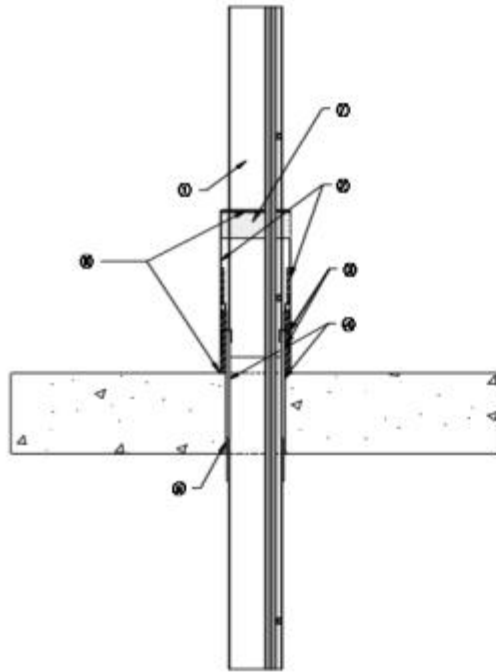
(수직 단면도 (A-A))
